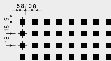
Регулярная квадратная перфорация 8/18 Q
