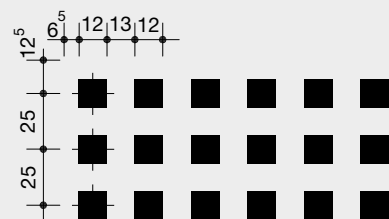
Регулярная квадратная перфорация 12/25 Q
