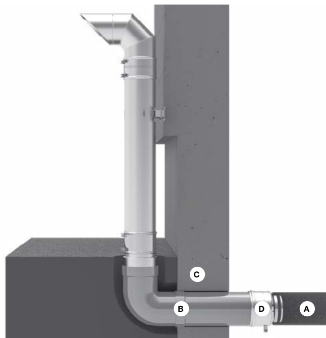
2 ComfoVent 180 System 2 Ниже уровня земли
